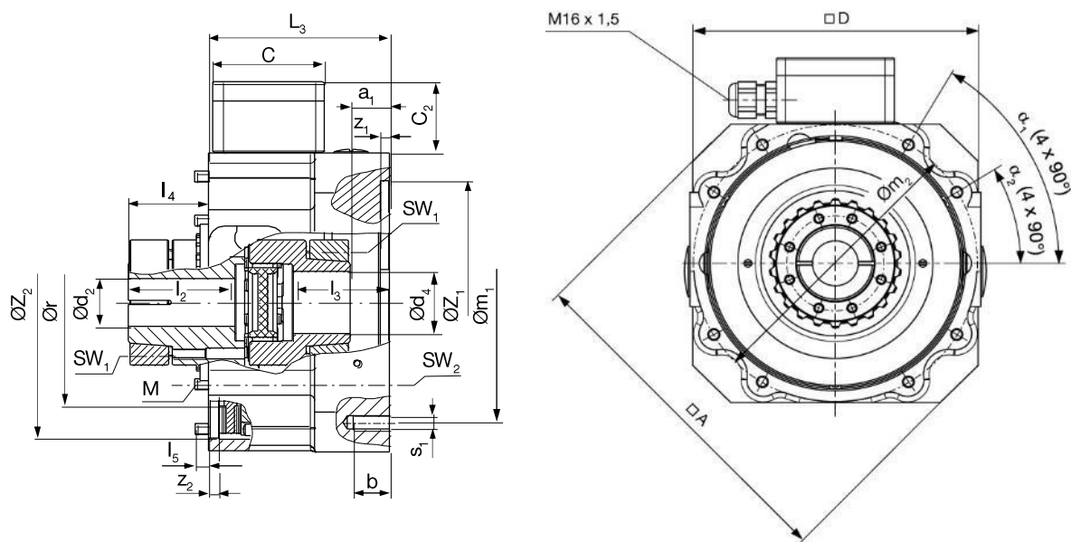
Fig. 16 Type 899.112. . . .
